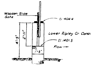
SECTION A-A 1" = 1'-0"
